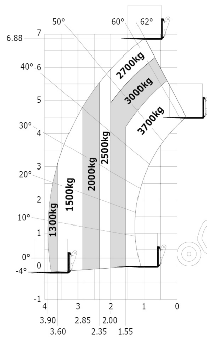
График для вездеходов (EN 1459 B)
